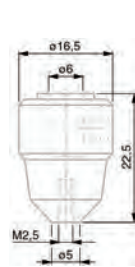
Axialer Messeinsatzhalter für Messeinsätze mit Gewinde M2,5
